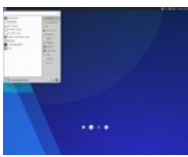
Xubuntu
