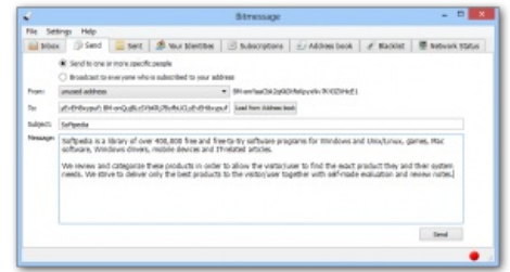
Пользовательский интерфейс
